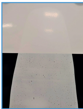
Fig. 5A White high gloss Acrylic-based enamel, without surface levelling additive Smalto acrilico bianco ad alta brillantezza, senza agente livellante
